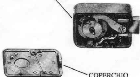
COPERCHIO
